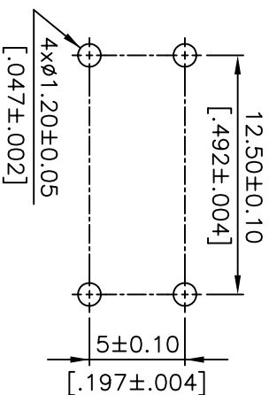
P.C.B. LAYOUT
