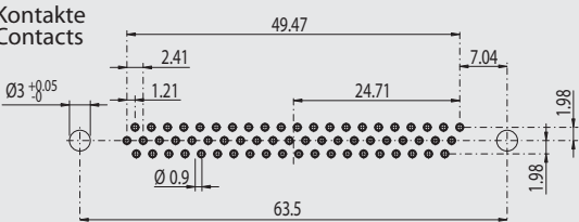
62 Kontakte Contacts
