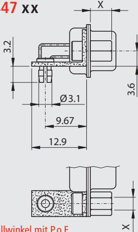
Metallwinkel mit P.o.F. Metal bracket with P.o.F.
