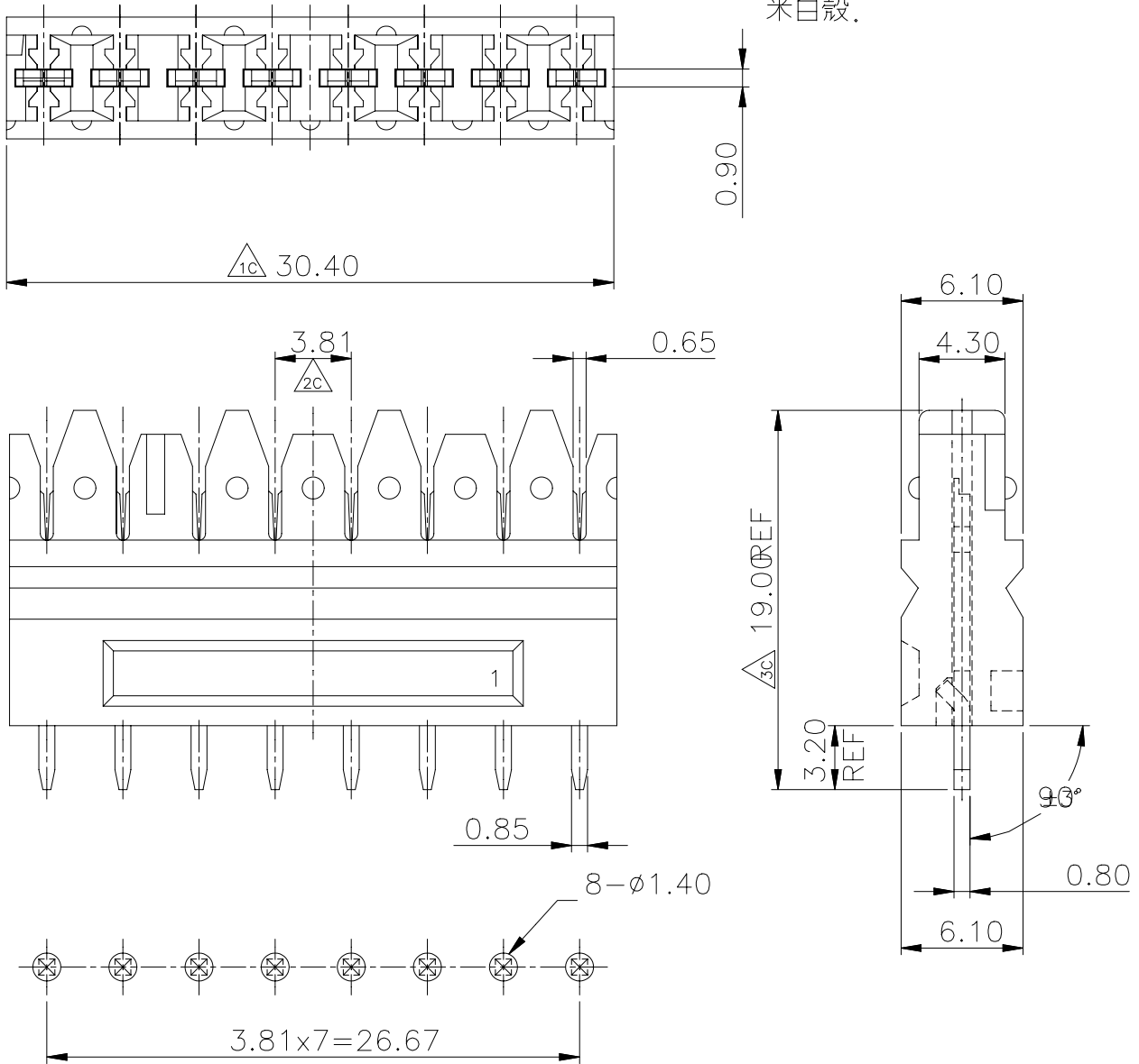
P.C.B LAYOUT
