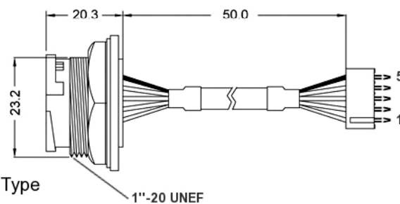
1''-20 UNEF
