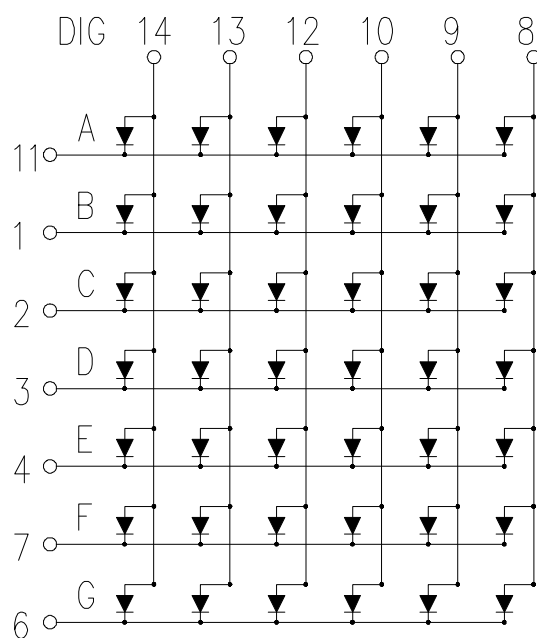
FYQ-3063Bx
