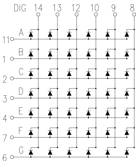
FYQ-3063Ax
