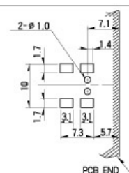
P.C.B DIMENSION
