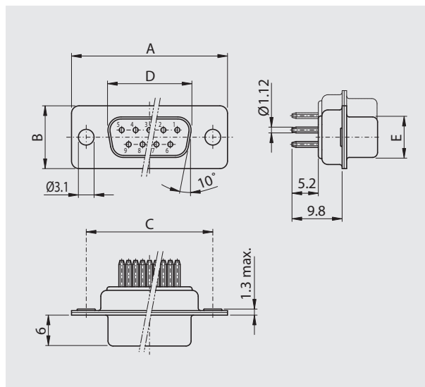
Buchsenleiste
