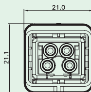
CABEL SIDE
