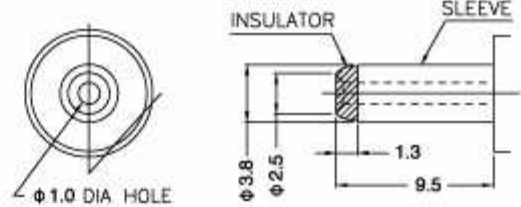
Fig. 4 MATCHING PLUG
