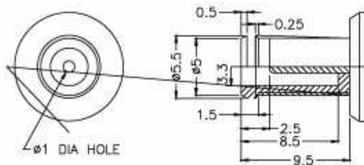
Fig. 5 MATCHING PLUG
