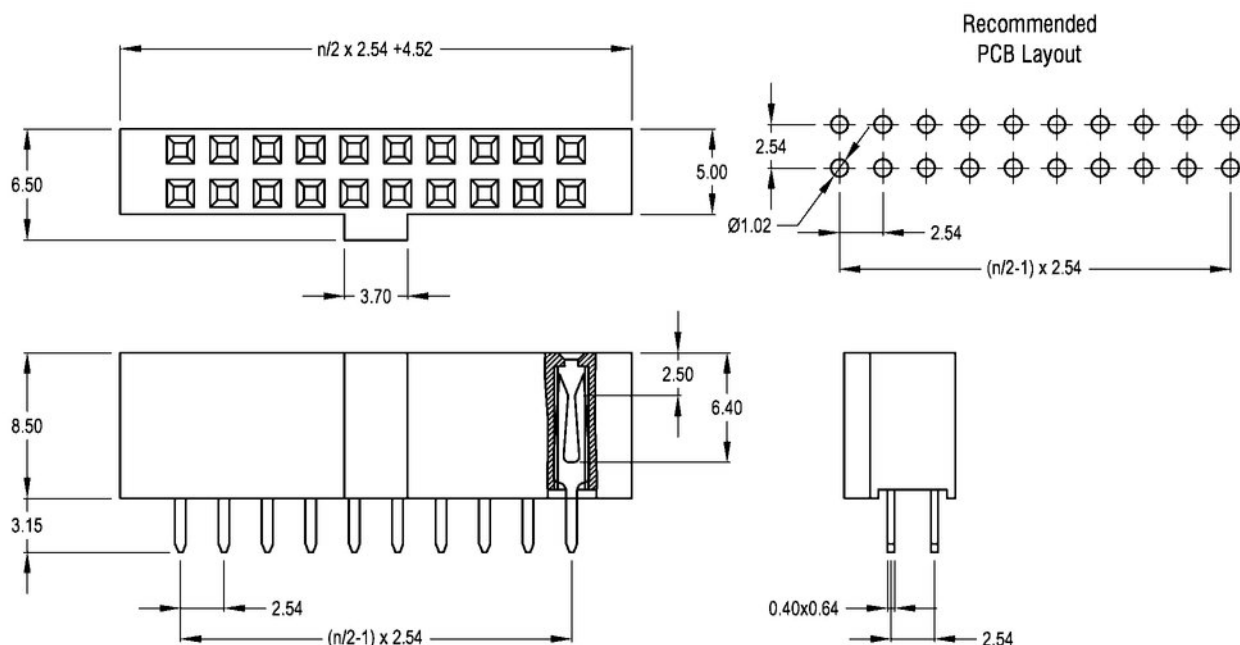
Gabelkontakte für Vierkantstifte 0,635mm. Fork contacts accept 0.635mm square pins. 137 1371
