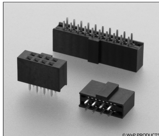
Gabelkontakte für Vierkantstifte 0,635mm. Fork contacts accept 0.635mm square pins. 137 1371
